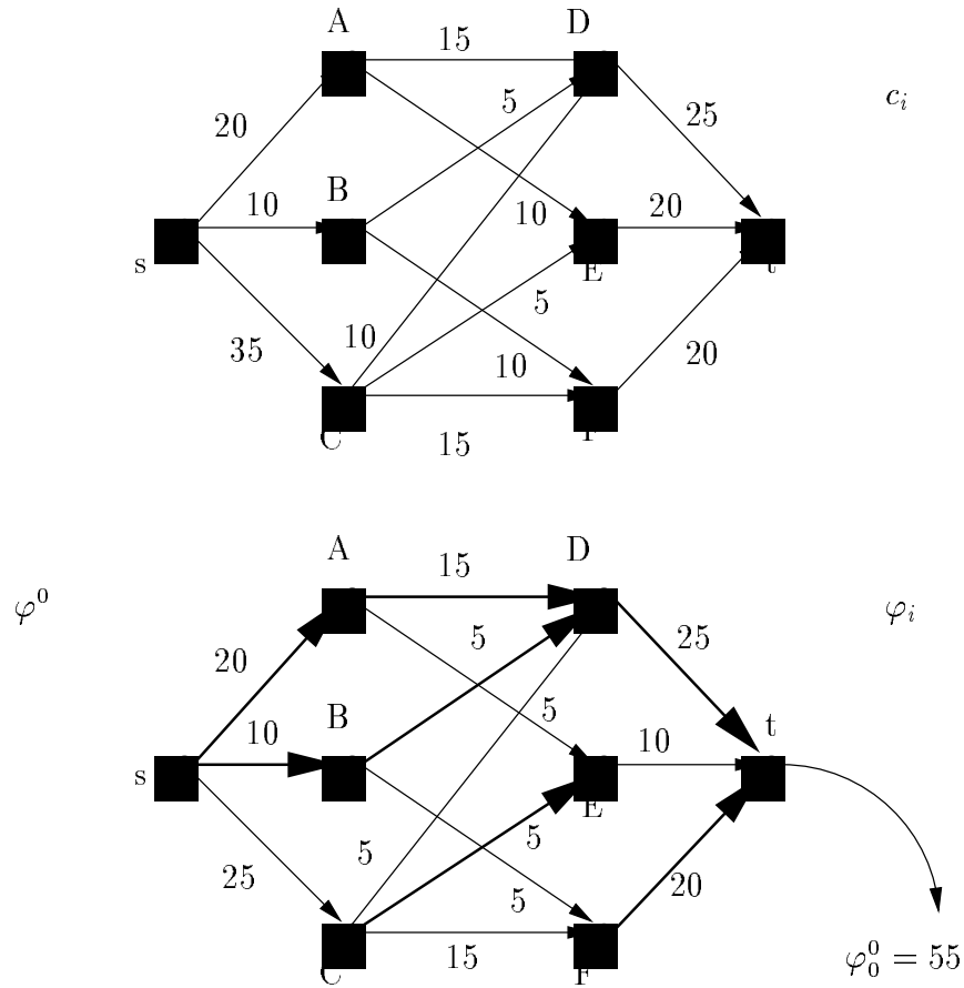
FIG. 4.4 – Procédure de Ford-Fulkerson à partir d'un flot complet
