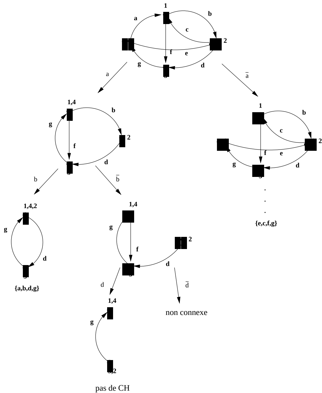
FIG. 3.5 – Enumération de circuits hamiltoniens
