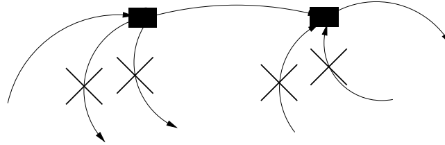
FIG. 3.4 – Procédure de simplification
