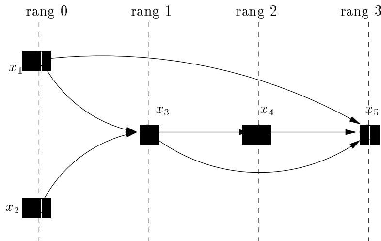
FIG. 1.17 – Décomposition en niveaux
