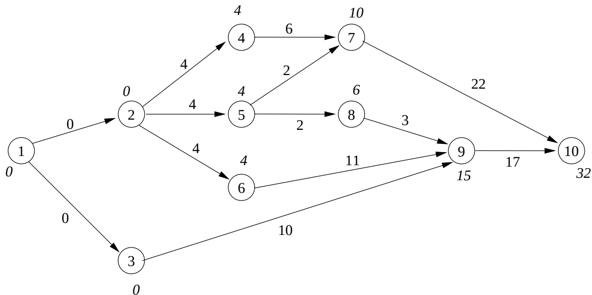
FIG. 1.18 – Réseau PERT
