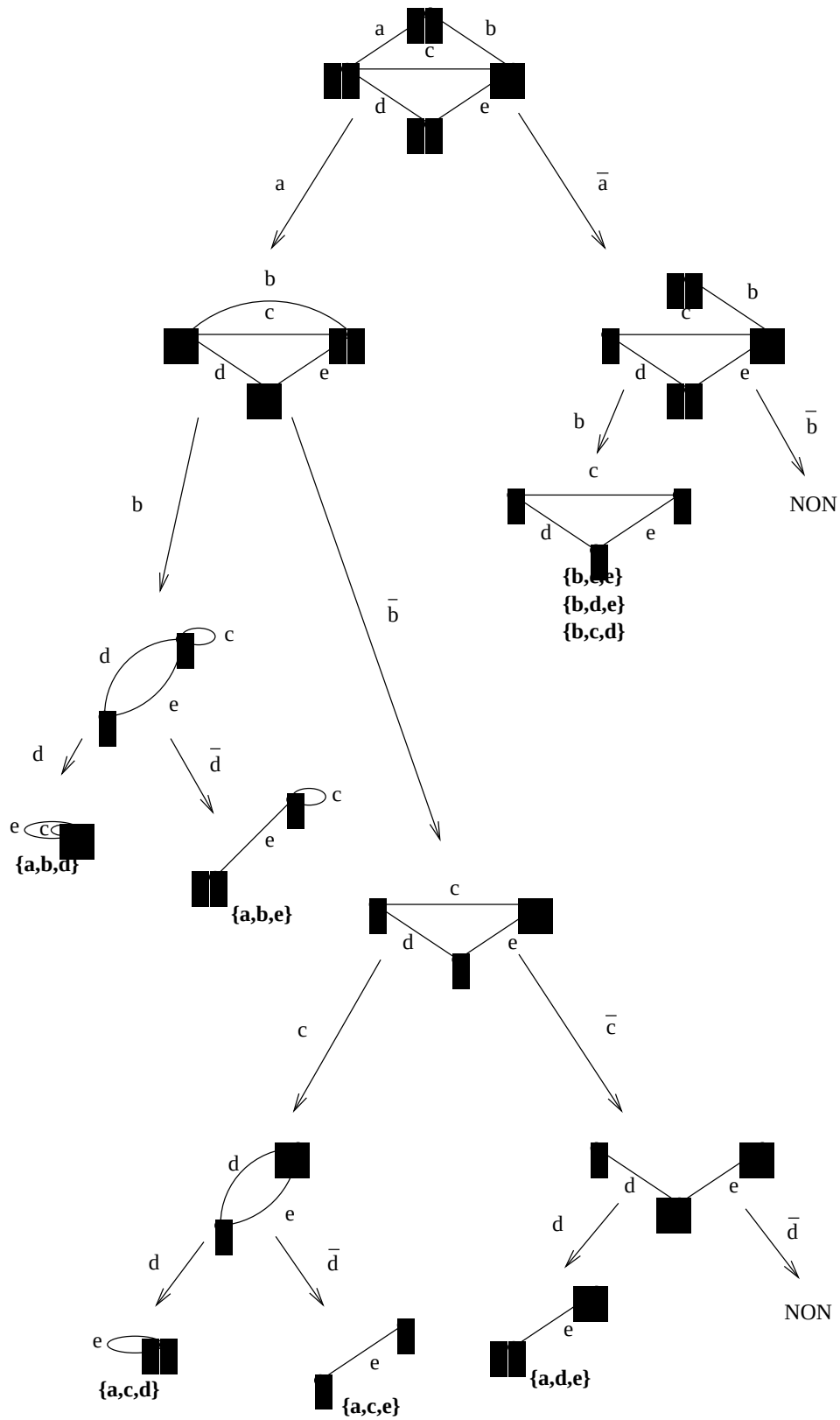
FIG. 3.6 – Enumération d'arbres
