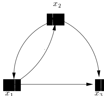
FIG. 1.5 – 1-graphe \equiv graphe
