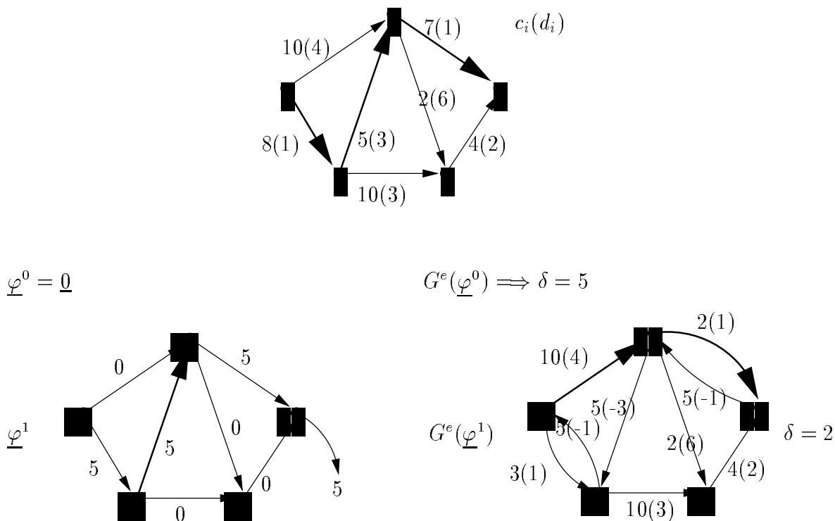
FIG. 4.6 – Procédure de Busacker-Gowen
