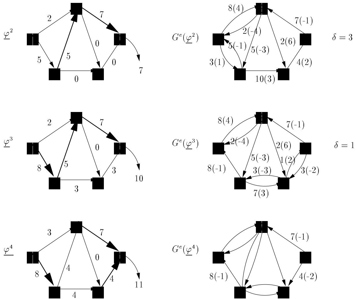
FIG. 4.7 – Flot maximum à coût minimum
