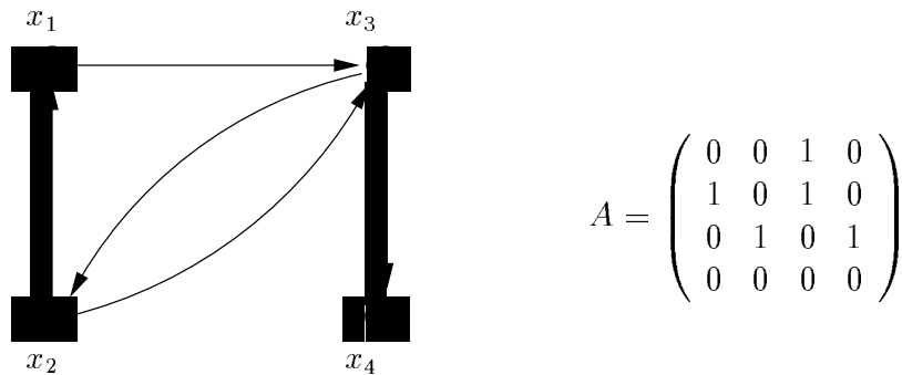
FIG. 3.1 – Existence de chemins
