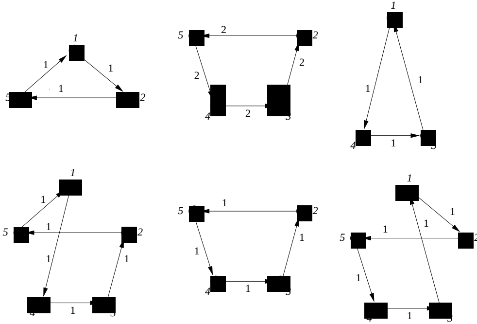
FIG. 4.2 – Flots cycliques élémentaires
