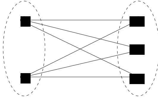
FIG. 1.19 – Grphe biparti complet K_{2,3}
