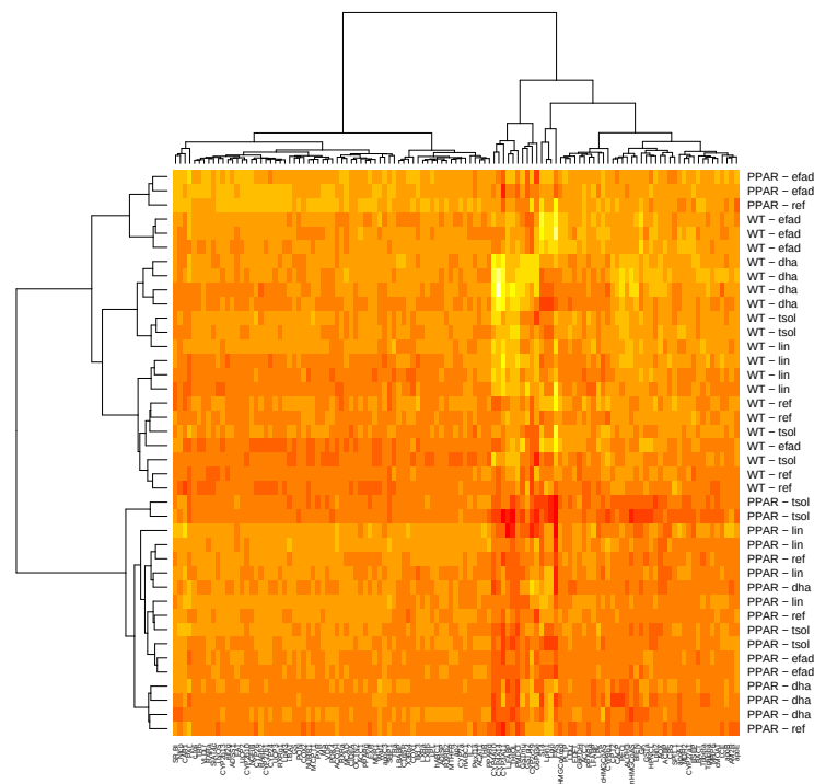
FIG. 5.8 – Souris : double classification ascendante hiérarchique des individus-souris et des variables-gènes selon la méthode de Ward, avec la distance euclidienne.
