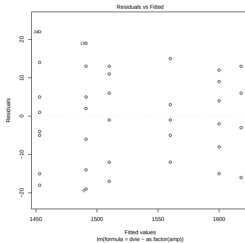
FIG. 8.1 – Données Ampoules : visualisation des résidus.
