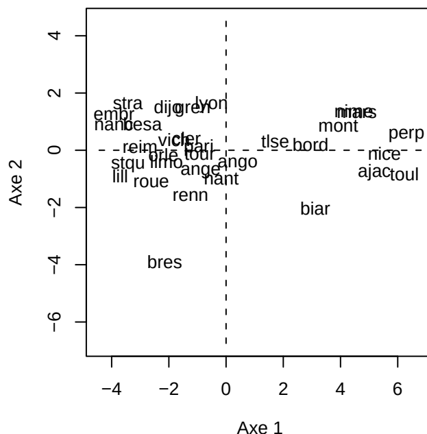
FIG. 3.4 – Températures : premier plan des individus.
