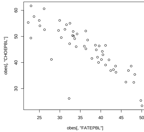
FIG. 2.5 – Obésité : Nuage de points illustrant la liaison linéaire entre deux variables biologiques.
