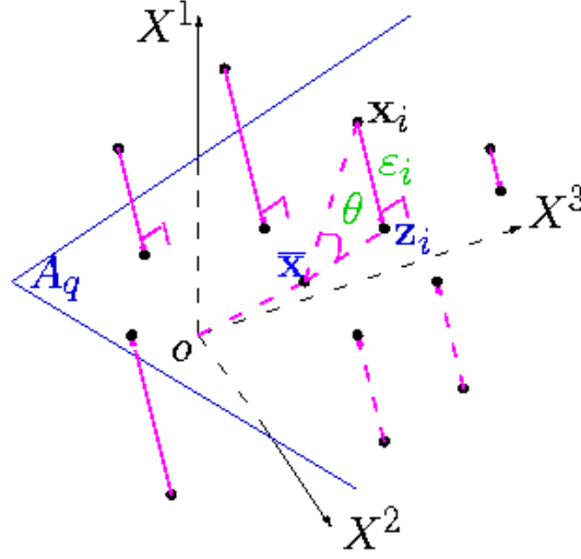
FIG. 3.3 – Principe de l'ACP dans l'espace des individus avec p = 3 .
