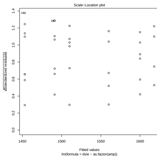
FIG. 8.3 – Données Ampoules : recherche de liaison moyenne-variance.
