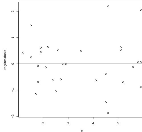
FIG. 7.4 – Données pH : plot des résidus vs variable explicative, pour le modèle (7.1).
