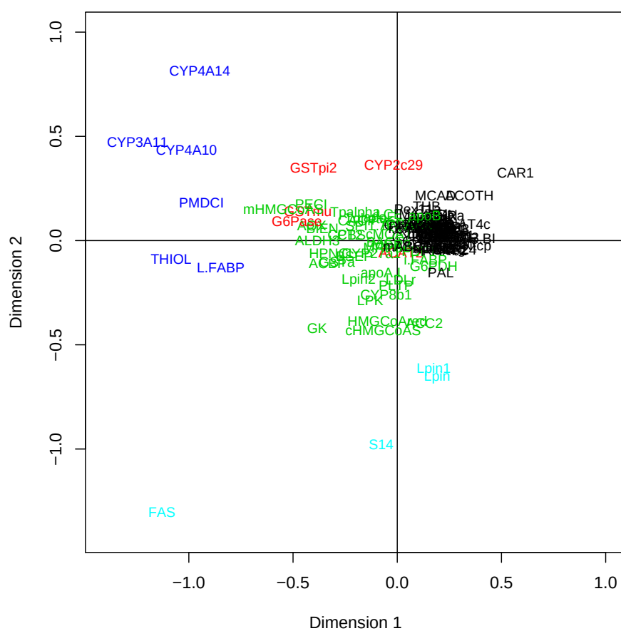
FIG. 5.10 – Souris : représentation par positionnement multidimensionnel (distance euclidienne) des 5 groupes issues de la classification hiérarchique des gènes.
