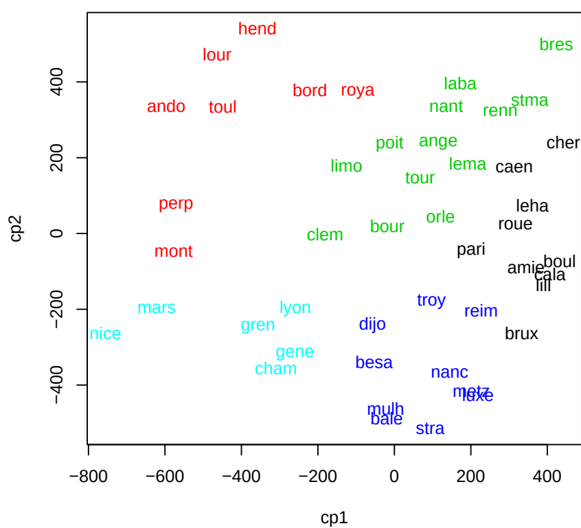
FIG. 5.3 – Villes : Représentation des classes (couleurs) obtenues par CAH dans les coordonnées du MDS.
