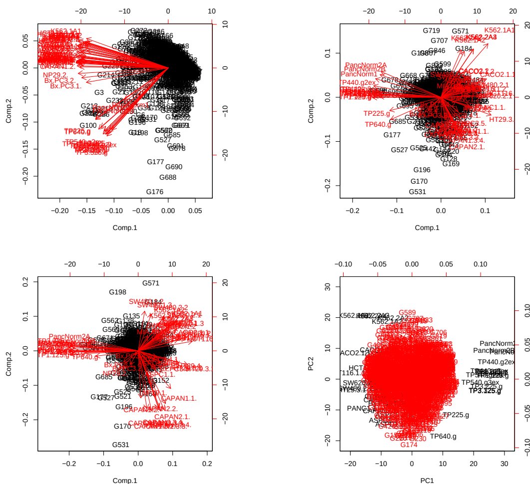
FIG. 3.10 – Pancréas : différentes options de l'ACP. a : gènes X tissus centrés. b : gènes centrés X tissus centrés. c : gènes centrés X tissus centrés réduits. d : tissus X gènes centrés réduits.
