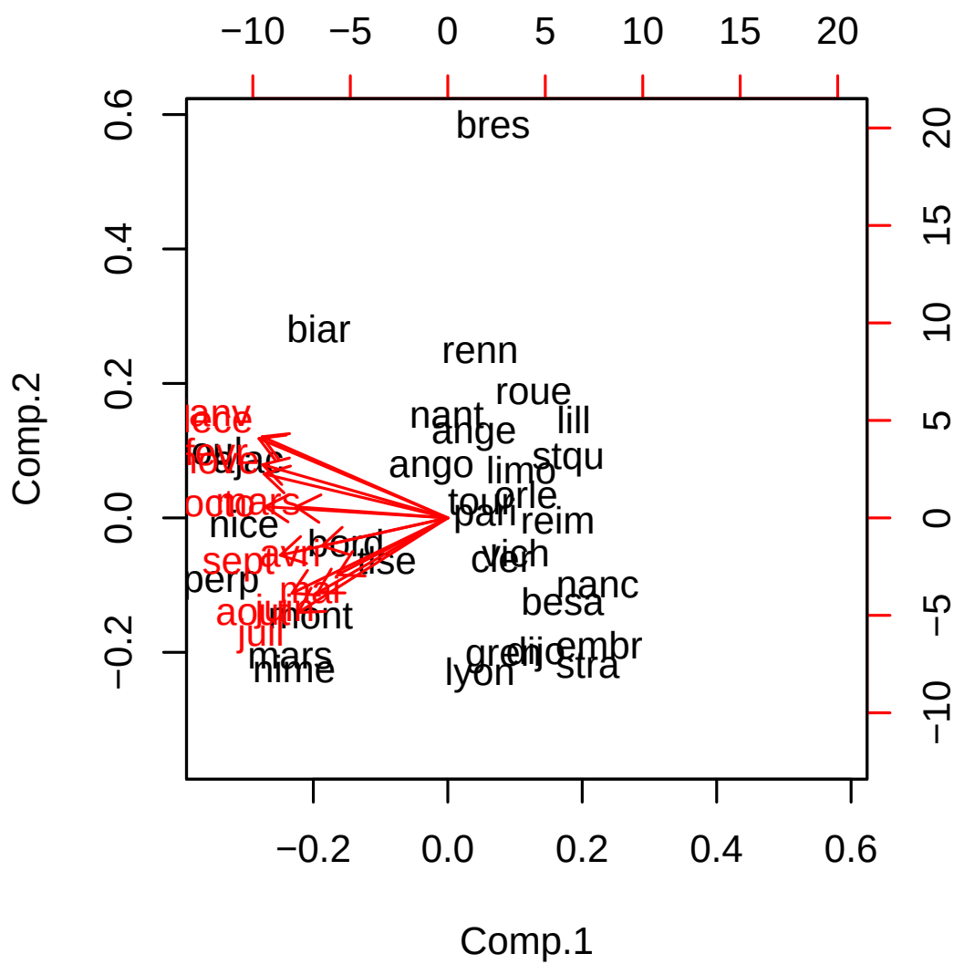
FIG. 3.6 – Températures : Représentation simultanée du premier plan.
