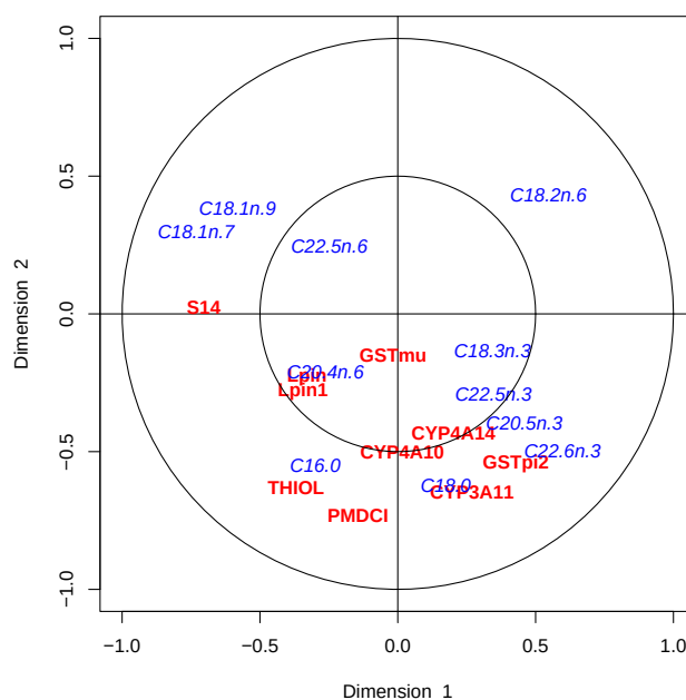
FIG. 6.2 – Souris : représentation des gènes (en rouge-gras) et des acides (en bleu-italique) dans le sous-espace des gènes.
