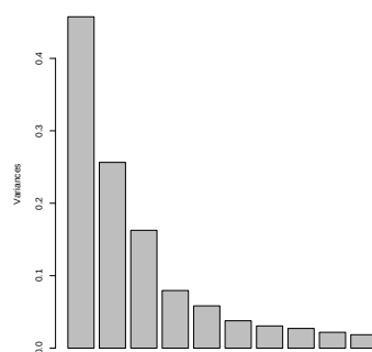
FIG. 3.14 – Souris : éboulis des dix premières valeurs propres de l'ACP.
