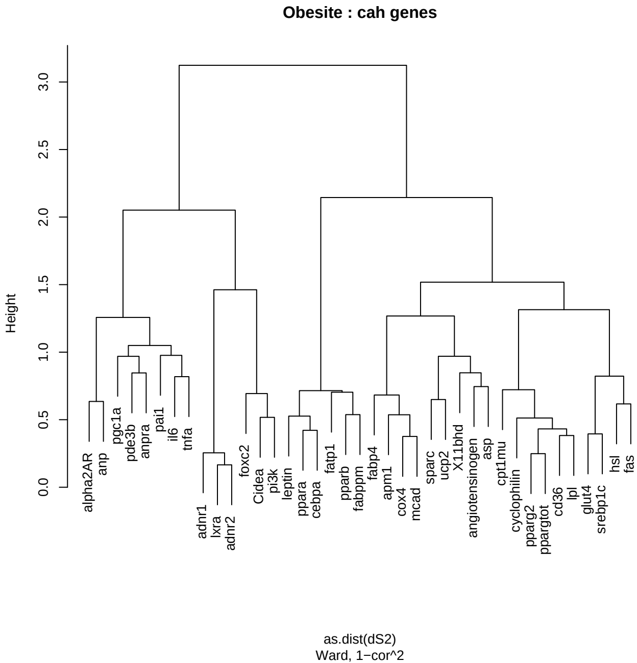
FIG. 5.7 – Obésité : Classification ascendante hiérarchique des gènes avec saut de Ward considérant le carré de la corrélation.
