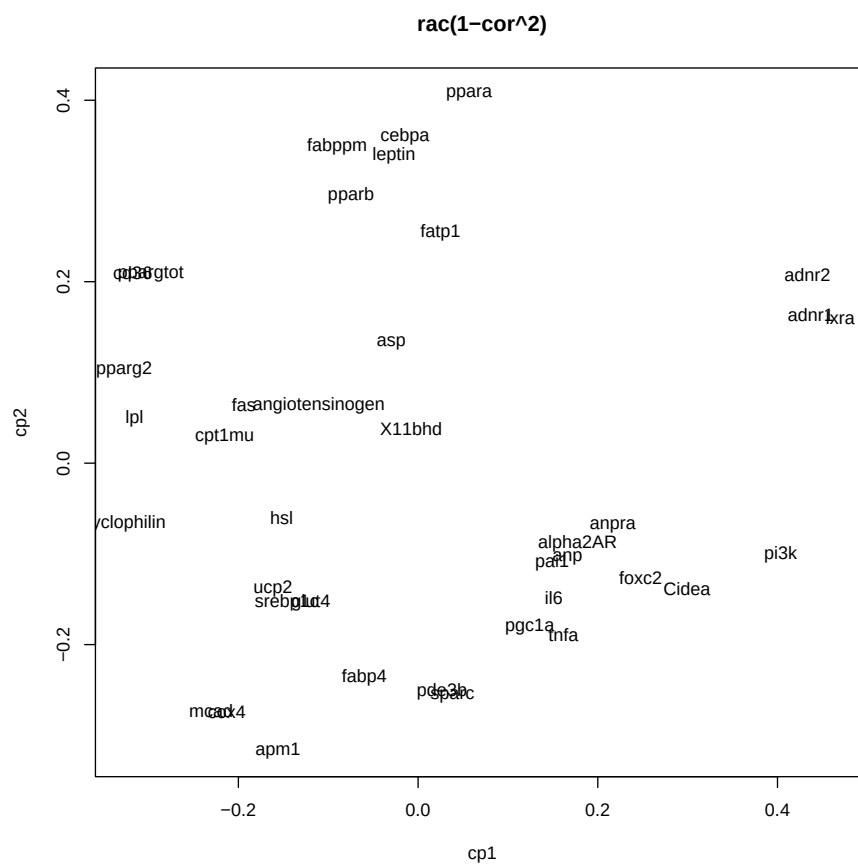
FIG. 4.4 – Obésité : représentation des gènes en fonction de leur proximité au sens de la corrélation au carré.
