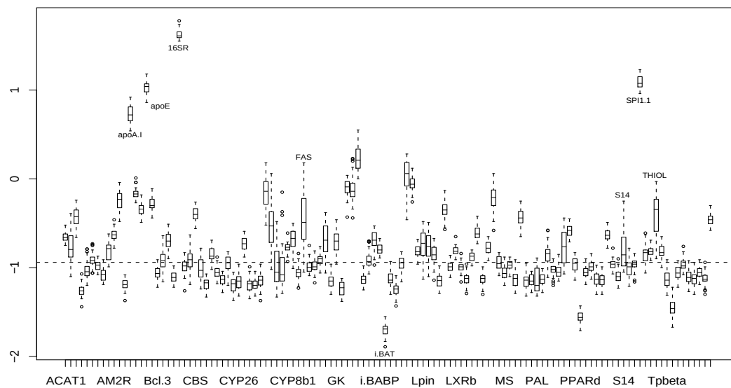
FIG. 2.9 – Souris : diagrammes en boîtes pour les 120 gènes. Quelques gènes particuliers ont été étiquetés.
