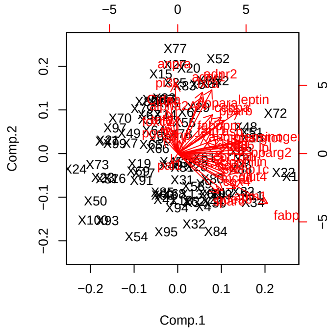
FIG. 4.2 – Obésité : Représentation du premier plan de l'analyse en composantes principales faisant apparaître un certain “effet taille”.
