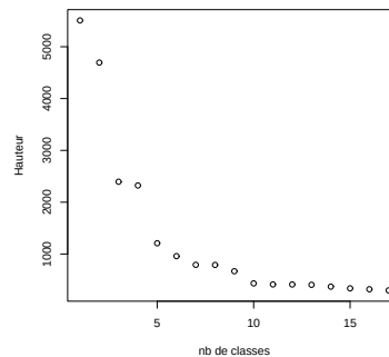
FIG. 5.1 – Villes : Décroissance de la variance interclasses à chaque regroupement dans le cas du saut de Ward.
