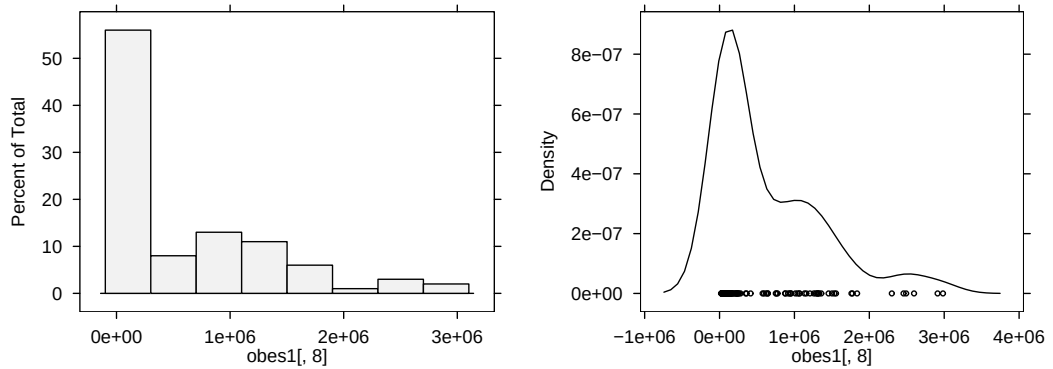
FIG. 2.3 – Obésité : Histogramme et estimation fonctionnelle par la méthode du noyau de la distribution de l'expression d'un gène.
