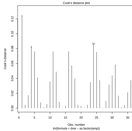
FIG. 8.4 – Données Ampoules : distance de Cook pour détection d'observations aberrantes.
