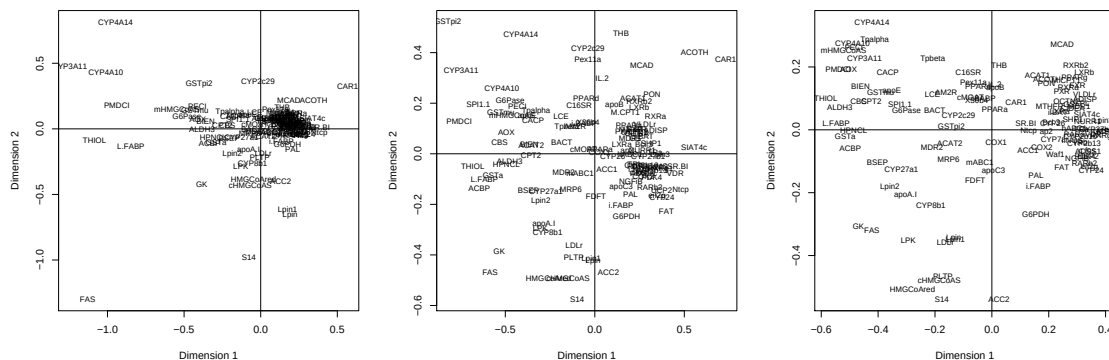
FIG. 4.6 – Souris : positionnement multidimensionnel des gènes sur les axes 1 et 2 selon 3 distances différentes : distance euclidienne ( d_1 à gauche), corrélation ( d_3 au centre), corrélation carrée ( d_2 à droite).
