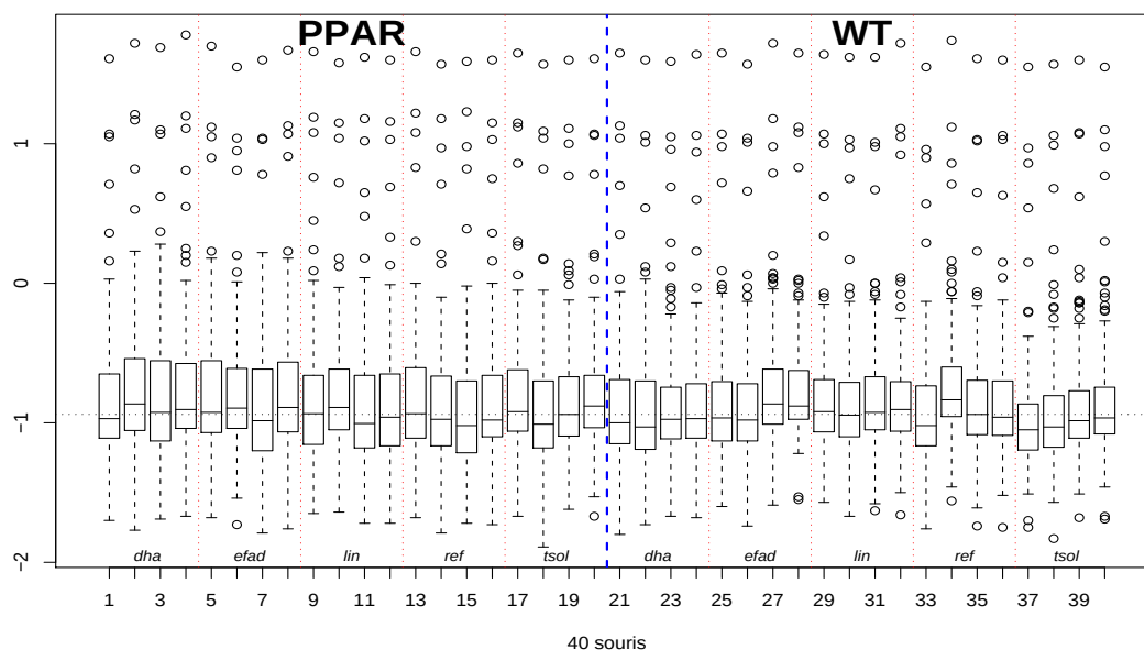
FIG. 2.8 – Souris : iagrammes en boîtes pour les 40 souris. La ligne verticale et épaisse sépare les souris selon leur génotype. Les lignes verticales et fines séparent les souris selon le régime qu'elles ont suivi. La ligne horizontale représente la médiane de l'ensemble des valeurs.
