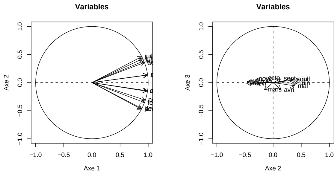
FIG. 3.5 – Températures : Premier et deuxième plan des variables.
