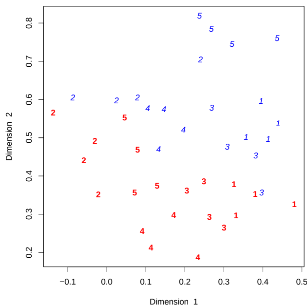
FIG. 6.1 – Souris : représentation des individus (souris) dans l'espace des gènes. Les WT sont en rouge-gras et les PPAR en bleu-italique ; les numéros correspondent aux régimes.
