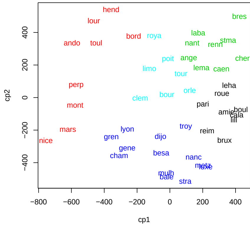
FIG. 5.4 – Villes : Représentation des classes (couleurs) obtenues par PAM dans les coordonnées du MDS.
