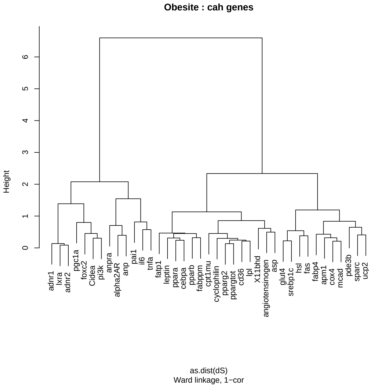
FIG. 5.6 – Obésité : Classification ascendante hiérarchique des gènes avec saut de Ward considérant la corrélation.
