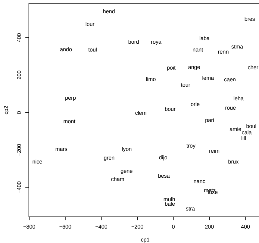
FIG. 4.1 – Villes : Positionnement de 47 villes à partir de la matrice de leurs distances kilométriques.
