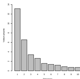
FIG. 5.9 – Souris : éboulis des valeurs propres pour le MDS de la matrice de distance euclidienne intergènes.
