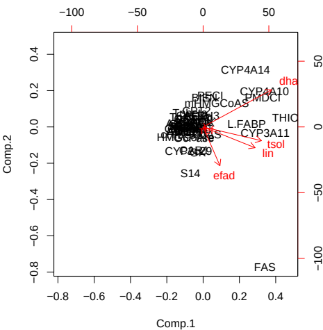
FIG. 8.5 – Souris : représentation sur le premier plan principal de l’ACP du logarithme des p -value des gènes différentiellement exprimés entre les deux génotypes à régime fixé.
