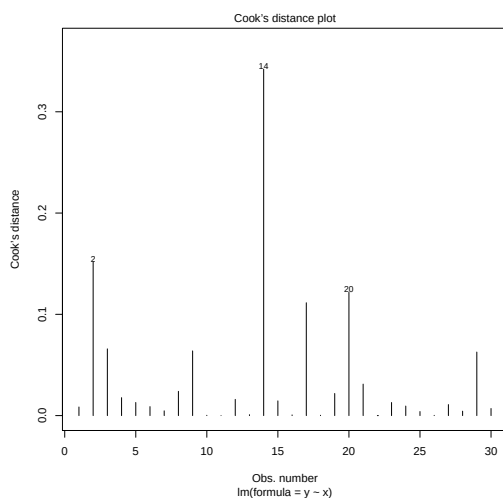
FIG. 7.6 – Distance de Cook pour le modèle (7.1) sur les données pH.
