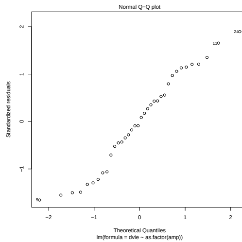
FIG. 8.2 – Données Ampoules : QQplot des résidus.
