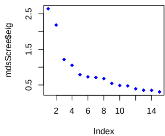
FIG. 4.3 – Obésité : Décroissance des valeurs propres et choix de la dimension de l'espace dans lequel rechercher une représentation euclidienne des gènes la plus conforme à leurs distances au sens de la corrélation au carré.
