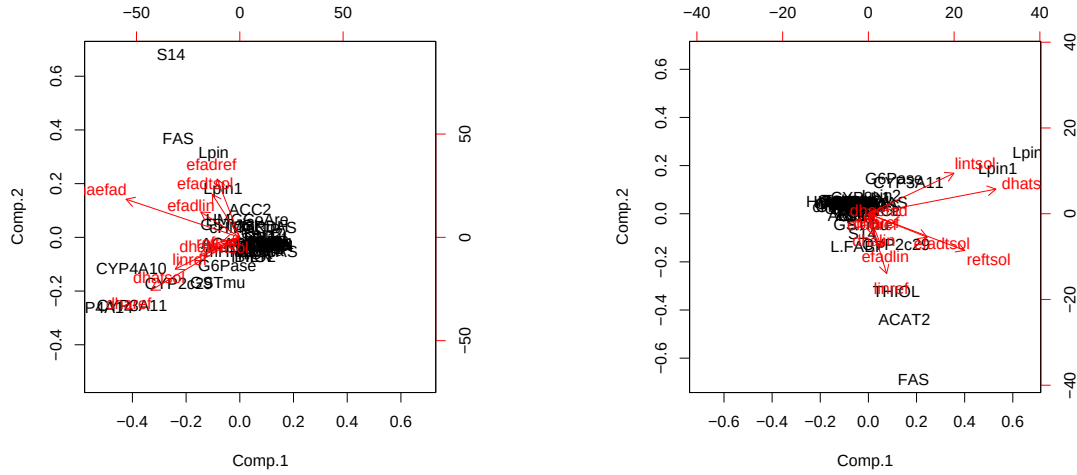
FIG. 8.6 – Souris : représentation sur le premier plan principal de l'ACP du logarithme des p -value des gènes différentiellement exprimés entre les régimes pour le génotype WT à gauche et PPAR à droite.
