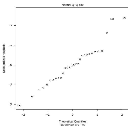
FIG. 7.5 – Données pH : QQplot du modèle (7.1).
