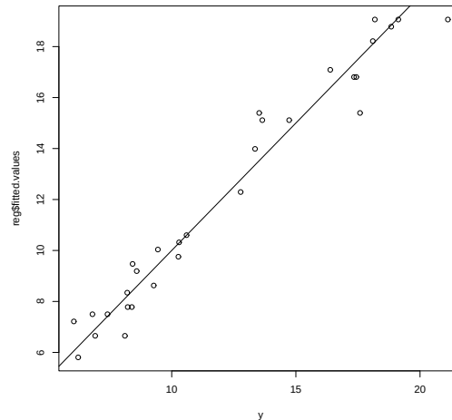
FIG. 7.2 – Données pH : droite de régression du modèle (7.1).
