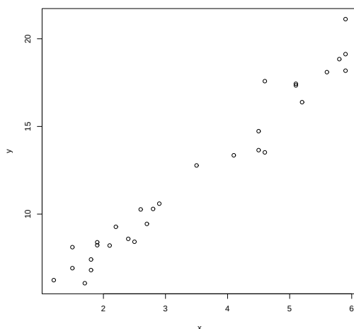
FIG. 7.1 – Données pH : le pH sanguin de 30 carpes vs. le pH ambiant.
