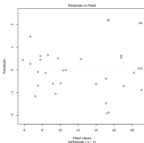
FIG. 7.3 – Données pH : plot des résidus vs valeurs ajustées, pour le modèle (7.1).
